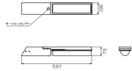
照明部 詳細図
