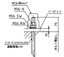
P部詳細図 (1:8)
