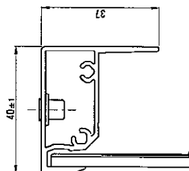
B-B' 断面 (S=1:1)
